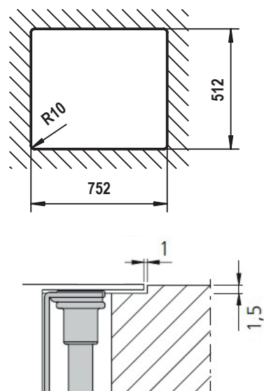
Installazione FILOTOP
